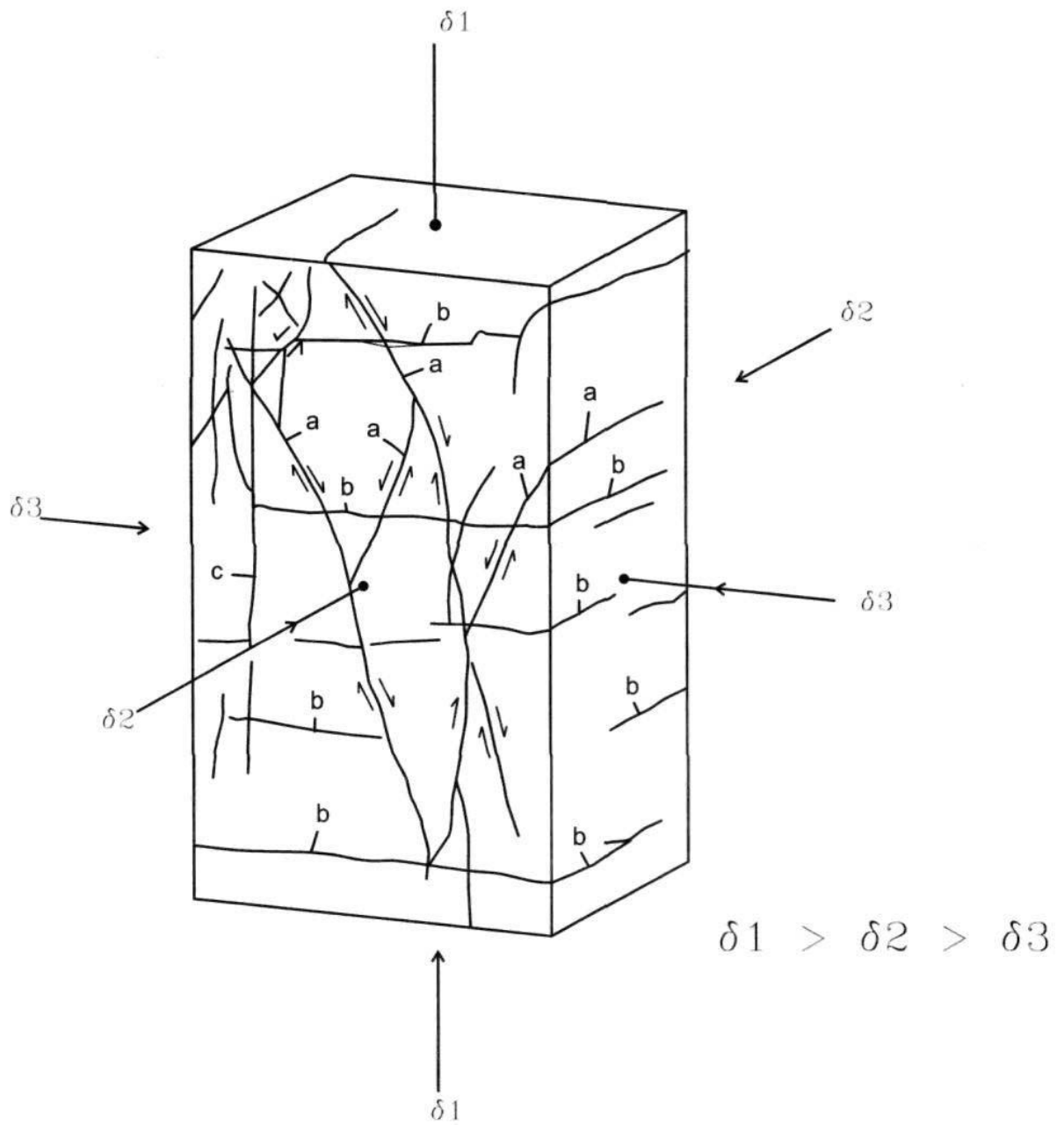
Figura A - Bloque de roca en ensayo de esfuerzos. Tres fuerzas compresivas afectan el bloque: sigma 1 ( \delta_1 ), mayor que sigma 2 ( \delta_2 ), mayor que sigma 3 ( \delta_3 ).
